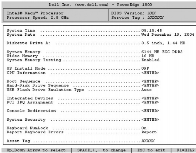
그림 3-1. 시스템 설치 프로그램 기본 화면
