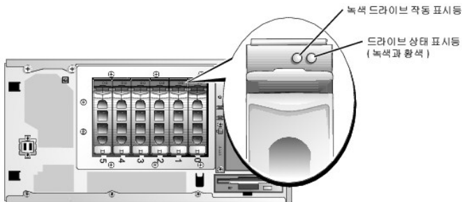
그림 1-3. SCSI 하드 드라이브 표시등
