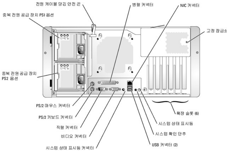
그림 1-4. 후면 패널 구조
